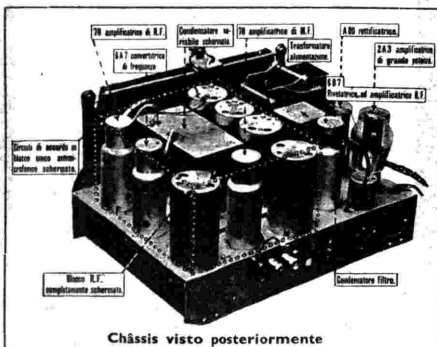
Chassis visto posteriormente
