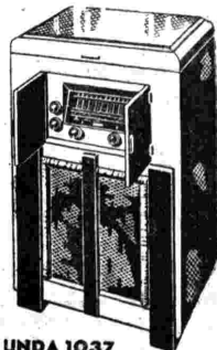
QUADRI UNDA 1037 Radiofonografo - Supereterod. 10 valvole - 4 campi d'onda - Selettività variabile - Potenza 15 W. Prezzo L. 4000
