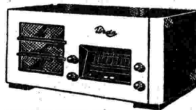
QUADRI UNDA 637 Supereterodina 6 valvole - 4 campi d'onda - Selettività variabile - Scale per ante brevetate - Potenza 3,5 W. Prezzo L. 1680
