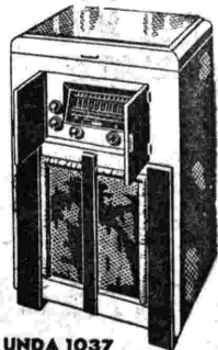
QUADRI UNDA 1037 Radiofonografo - Supereterod. 10 valvole - 4 campi d'onda - Selettività variabile - Potenza 15 W. Prezzo L. 4000
