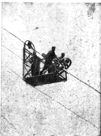
Carrello scorrevole sugli stralli per la manutenzione dell'antenna.
