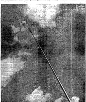
L'antenna autotransmissante del trasmettitore di Milano III.
