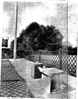
Un dettaglio dell'antenna autoirradiante e della linea di trasmissione.
