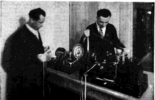
Apparecchi di registrazione impiegati nelle misure di frequenza.
