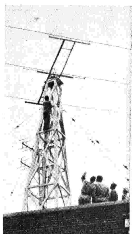
Un nuovo tipo di antenna a raggio rotante di costruzione americana per il collegamento con gli aerei in volo.
