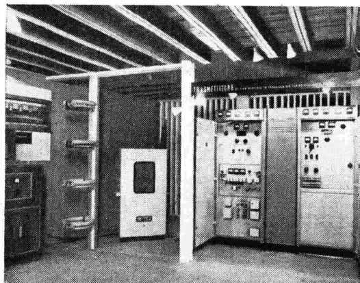
Impianti della RAI alla Mostra: (da sinistra) il «magnetofono», i quattro elementi «radianti» dell'antenna direttiva, un apparecchio ricevente ad alta fedeltà, il trasmettitore ad onde ultracorte con modulazione di frequenza.
