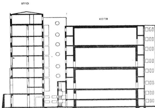
SEZIONE VERTICALE DEL NUOVO PALAZZO DELLA RADIO DI MILANO. — Lato Uffici, dall'alto: Sala amplificatori, sale tecniche di controllo e smistamento programmi, uffici sezione tecnica, uffici sezione programmi, uffici della Direzione della sede, uffici della Sezione Propaganda e Sviluppo, salone del pubblico, sotterranei per i servizi accessori, Lato Auditori, dall'alto: Complessi prosa, complessi musica, complessi televisione, seminterrati e sotterranei per i servizi accessori.
