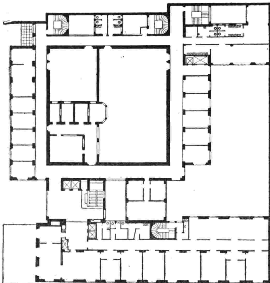
SEZIONE ORIZZONTALE AL PIANO DELLA MUSICA DEL NUOVO PALAZZO DELLA RADIO A MILANO. — Al centro: L'Auditorio grande e l'Auditorio medio con le relative sale regia e salette annunciatori; attorno ad essi i vari locali accessori e di servizio. In basso: L'ala degli Uffici della Direzione Compartmentale di Milano.
