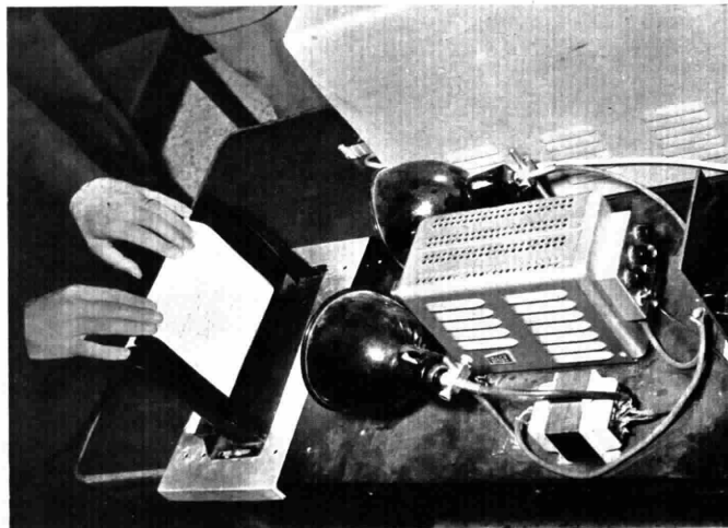
Il «vidicon» si compone di un piccolo impianto trasmettente e di uno ricevente. Nella fotografia, la telecamera installata in redazione mentre sta riprendendo un dattiloscritto (Foto Luxardo)
