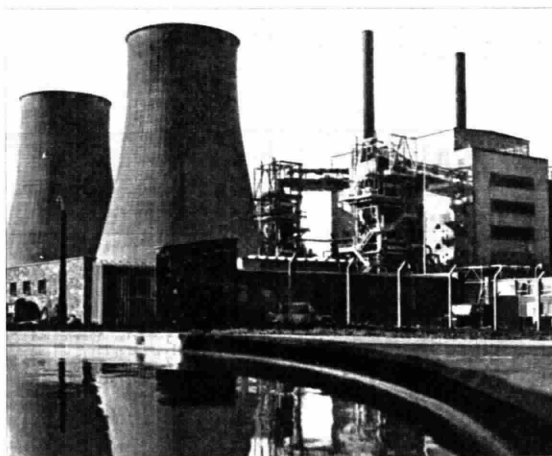
Calder Hall: la prima centrale elettronucleare commerciale costruita nel mondo. Entro il 1965 la Gran Bretagna disporrà di sette centrali elettronucleari con una potenza complessiva installata di 6000 MW (megawatt)
