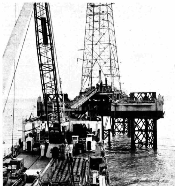
Il «pozzo 28» a due chilometri e mezzo dalla costa: è costituito dallo «Scarabeo», il pontone che regge la grande sonda, e dalla nave-appoggio «Saipem»
