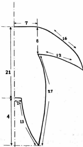
Questa è la mezza sagoma per « Crispino »: i numeri corrispondono a centimetri
