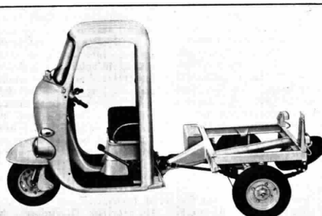
Vista del mototelaio Lambro 550 su cui vengono montate le elaborazioni speciali (portabidoni, scala estensibile, servizio antincendio, motocisterna, motor-riciclaw e tante altre). Sono vari: il telaio in tubo d'acciaio e il telaio posteriore in travi a C. Caratteristiche tecniche: cilindrata 198 cc - potenza max 9,2 cv - giri minuto 4800 - rapporto compressione 7:1 - cambio 4 marce + 1 a - consumo 11,6/100 km - velocità max effettiva 58,3 km/h - velocità max a pieno carico 53,7 km/h - miscela 4 % - portata max 550 kg (cassone aperto) 540 kg (cassone chiuso).
