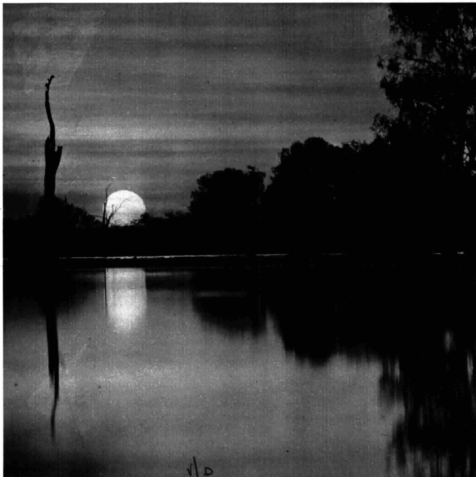
L'acqua fu la culla della vita. In lagune stagnanti come questa alcune sostanze chimiche, sotto lo stimolo di cariche elettriche e radiazioni solari, si unirono in molecole complesse dando luogo alle prime forme di vita terrestre
