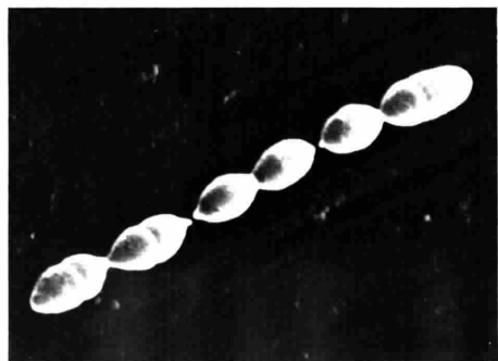
A fortissimo ingrandimento, ecco uno dei nostri invisibili nemici, lo Streptococcus pyogenes
