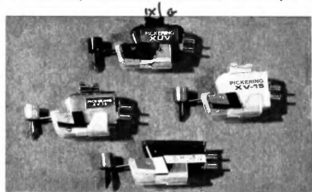
Un gruppo di testine della Pickering. In alto la XV/4500 Q con equipaggio mobile in lega di cobalto che ha una massa ridotta a 1/10 del normale, adatta alla riproduzione stereo e quadrifonica con puntina di taglio speciale
