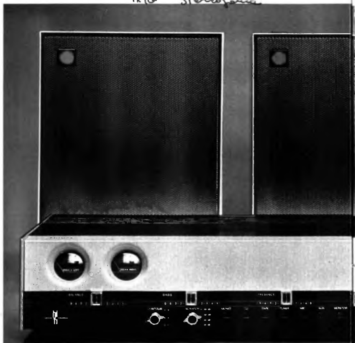
PHILIPS RH551 — Questo preamplificatore è stato costruito appositamente per pilotare le casse acustiche attive « Motional Feedback » (che appaiono anche nella foto) che contengono, oltre agli altoparlanti, anche gli amplificatori di potenza. Esso è però adattabile anche alla maggior parte degli amplificatori finali di potenza in commercio. La tensione di uscita è di 1,1 Volt a 1 kHz, la distorsione è contenuta nello 0,09 %: un valore senz'altro ottimo
