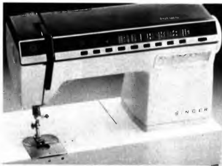
Eccola! Futura della Singer, la prima macchina per cucire a programmazione elettronica.
