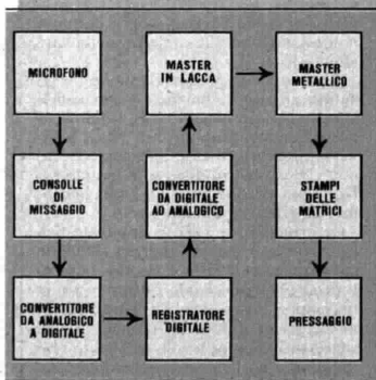
DIAGRAMMA A BLOCCHI DEL PROCESSO DI REGISTRAZIONE DIGITALE
