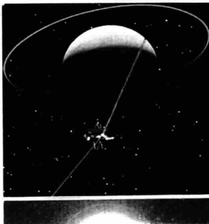
Nella foto: la navicella spaziale nel punto più vicino a Urano, in una immagine creata dal computer
